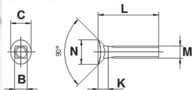
Култиваторен болт с елипсоидна глава
